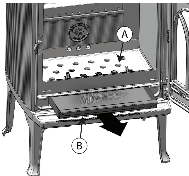
Kuva 14 Tuhkaritilä
