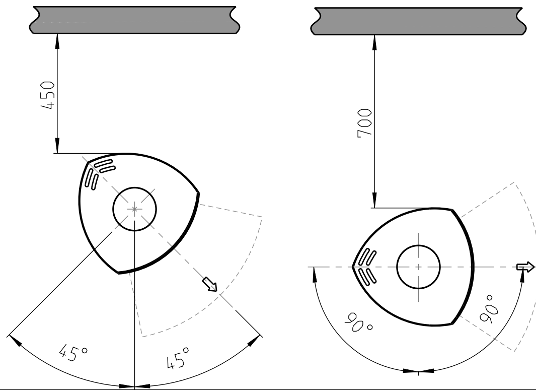
Min. avstand til brennbar vegg med dreibar søyle
