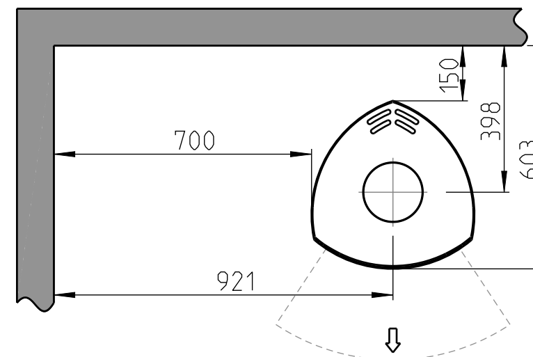
Min. avstand til brennbar vegg
