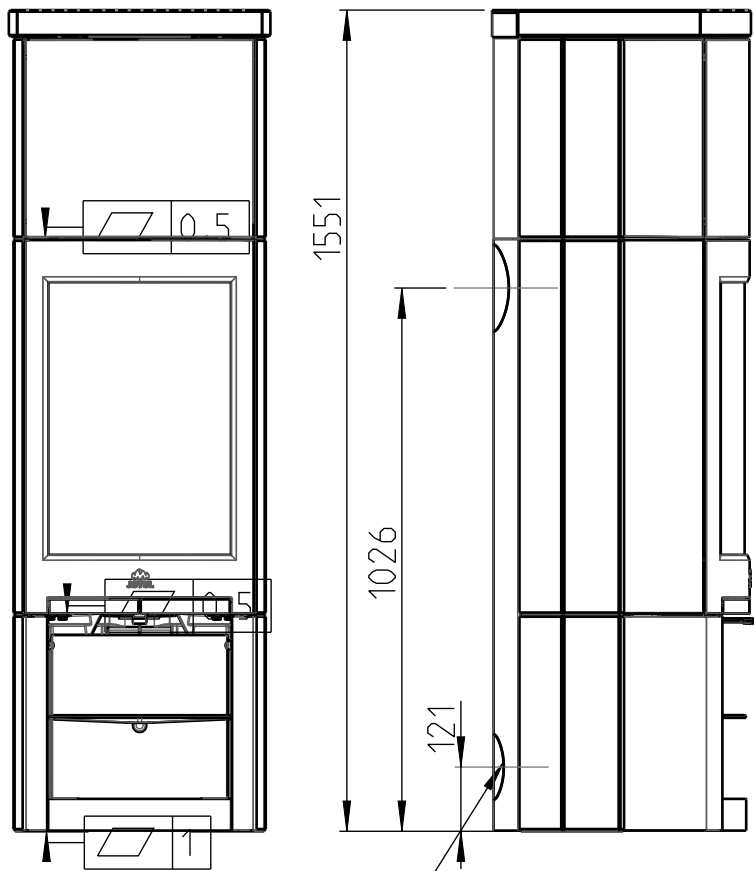
Jøtul F 367 Advance med High Top
