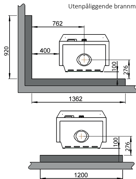
Utenpåliggende brannmur
