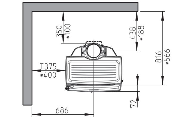
Min. avstand til brennbar vegg
