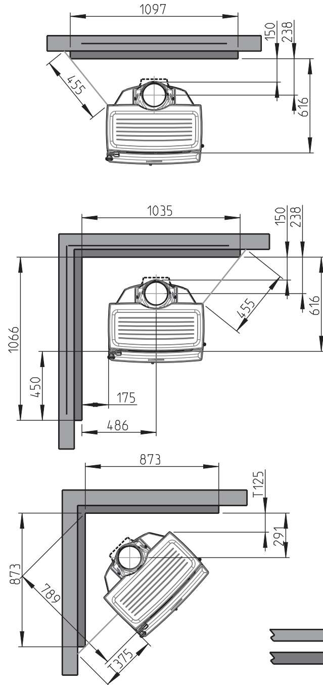
Utenpåliggende brannmur
