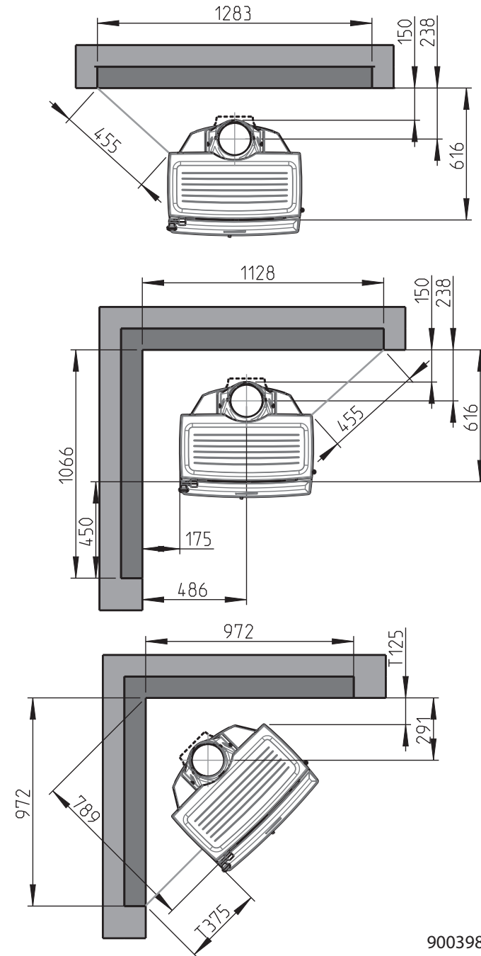
Innfelt brannmur
