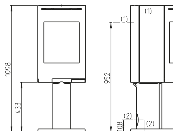
Jøtul F 136 med søyle og uten sideglass
