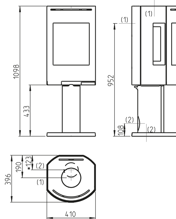
Jøtul F 137 Med søyle og uten sideglass
