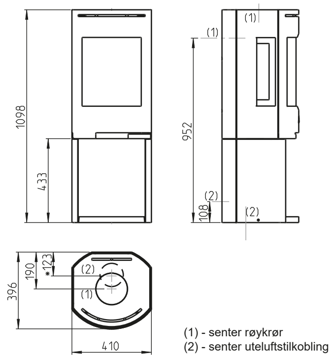
Jøtul F 135 med sokkel og sideglass
