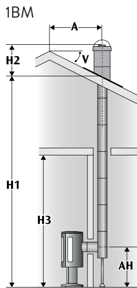
Bakmontering gjennom skillevegg.
