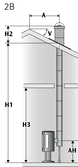
Bakmontert direkte bak ildsted. Helisolert pipe.
