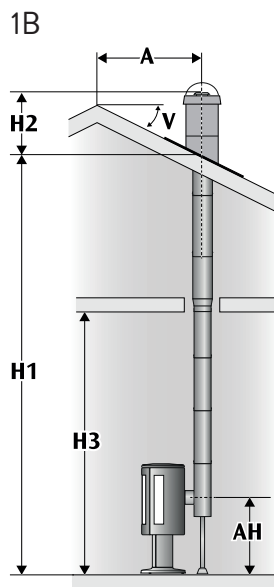
Bakmontering direkte bak ildsted. Halisolert startør med overgang skjult i bjelkelag.
