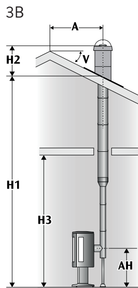
Bakmontering direkte bak ildsted. Uisolert startør.
