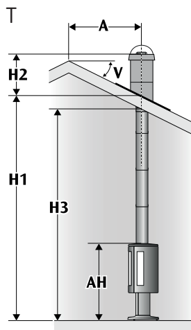
Toppmontert halisolert
