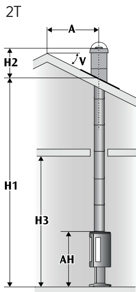
Helisolert pipe.
