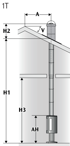
Halisolert startør med overgang skjult i bjelkelag.
