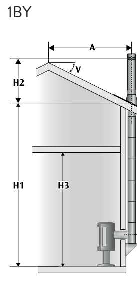
Bakmontering gjennom yttervegg.
