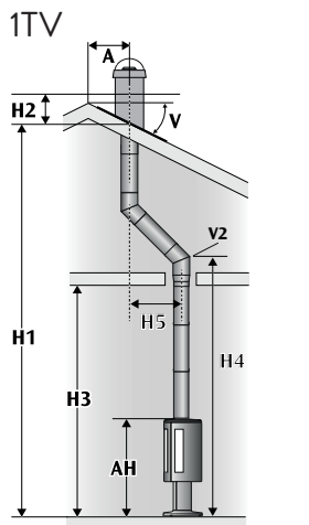
Toppmontering med halisolert startør og senterforskyvning.
