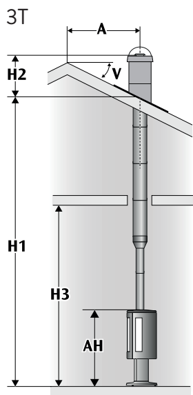
Uisolert startør.
